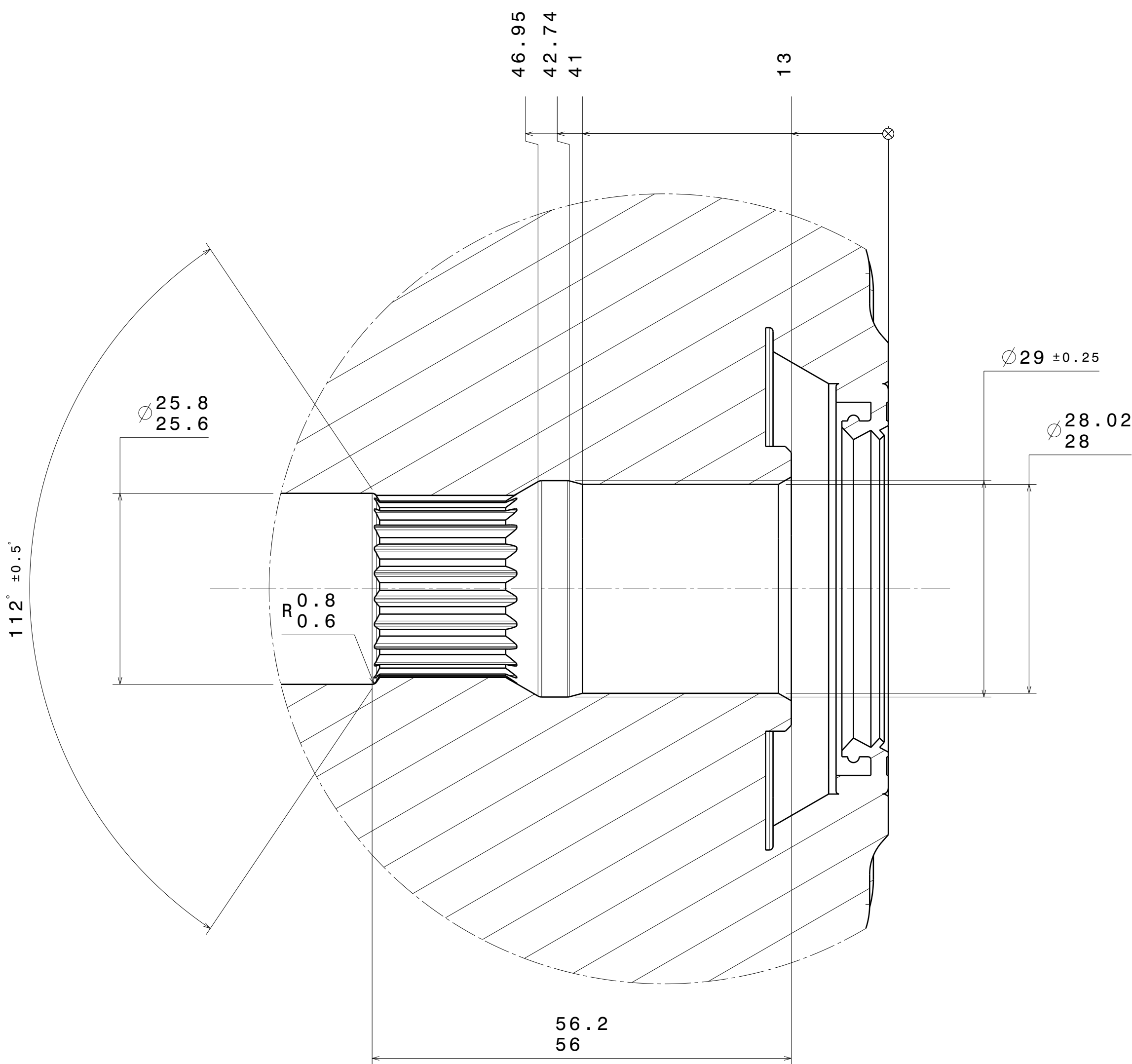
Section view A-A Scale: 2:1
